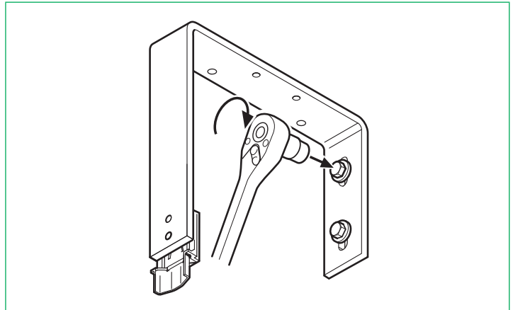
＜マウンティングブラケット取り付けイメージ＞
